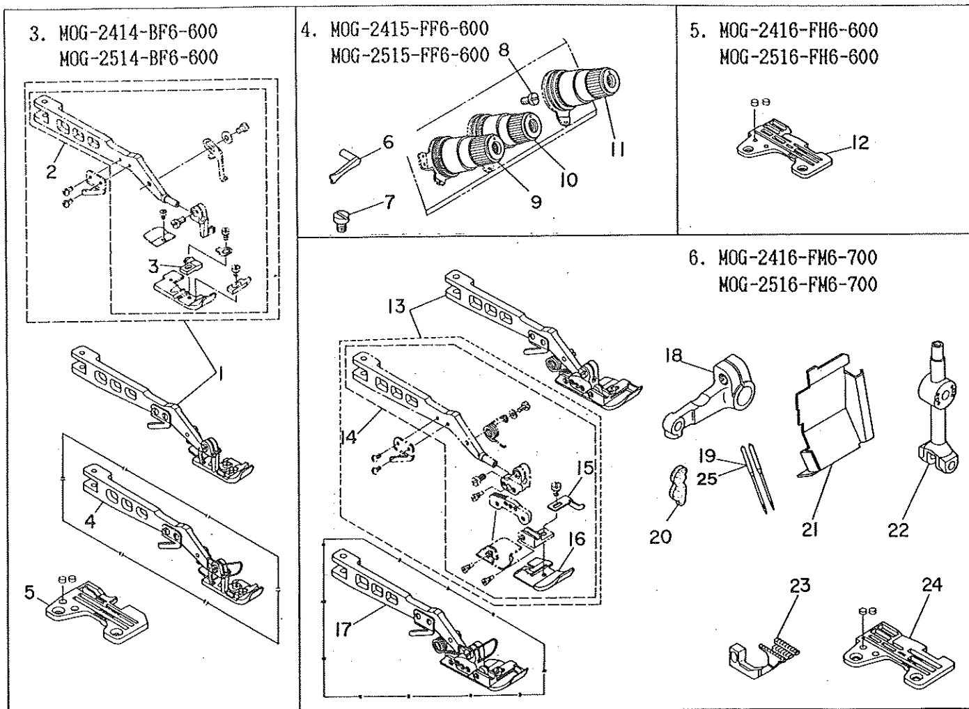
3. MOG-2414-BF6-600 MOG-2514-BF6-600
